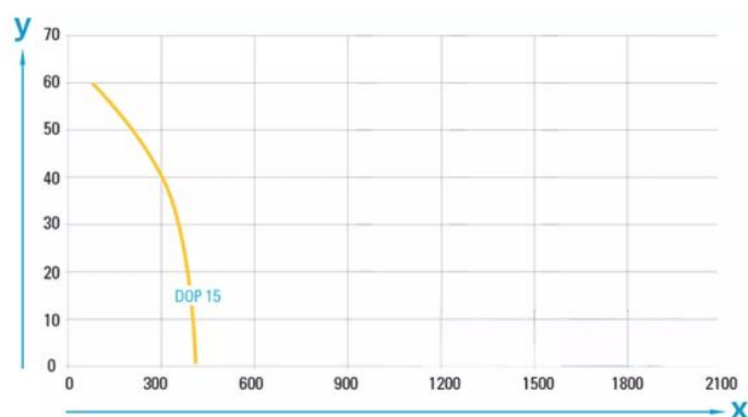
Diagramma di flusso per pompe pneumatiche DOP per fluidi inquinati ad alta viscosità
