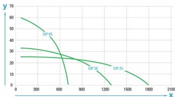
Diagramma di flusso per pompe pneumatiche DIP per fluidi puliti a bassa viscosità
